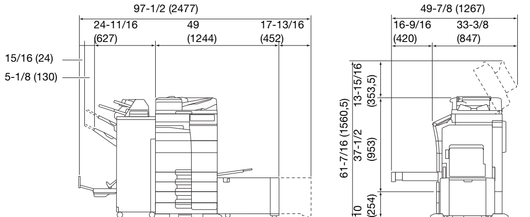
bizhub C658/C558/C458 + PC-215 + FS-537+ SD-512 + RU-513 + PI-507 + LU-207 Μονάδα: ίντσα (mm)
