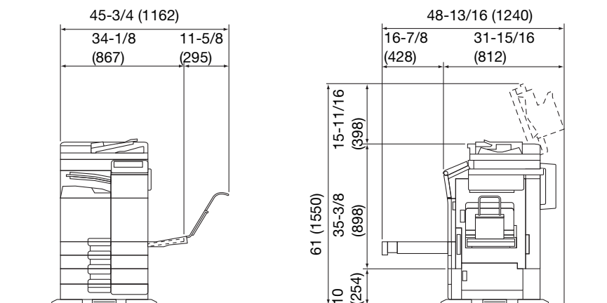
bizhub C368/C308/C258 + DF-629 + PC-210 + JS-506 + MK-730 + CU-101 + MK-745 Μονάδα: ίντσα (mm)
