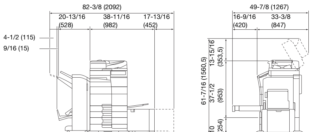
bizhub C658/C558/C458 + PC-215 + FS-536 + SD-511 + RU-513 + PI-507 + LU-302 Μονάδα: ίντσα (mm)
